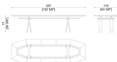
SC1013/B Two trestle table Tavolo con due basi
