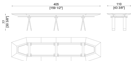
SC1013/A Three trestle table Tavolo con tre basi
