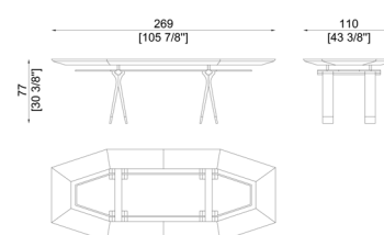
SC1013/C Two trestle table Tavolo con due basi
