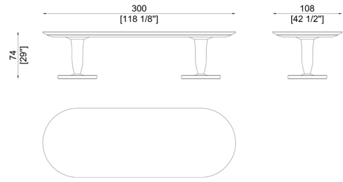
SC1029 Elliptical table with two bases Tavolo ovale con due basi
