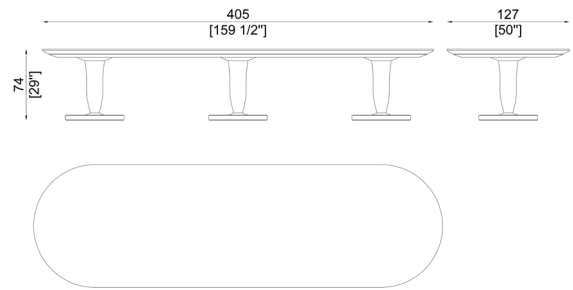
SC1029/B Elliptical table with three bases Tavolo ovale con tre basi
